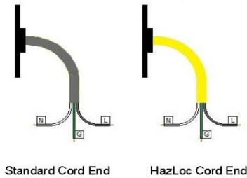
Standard Cord End HazLoc Cord End
